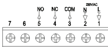
Šema povezivanja
